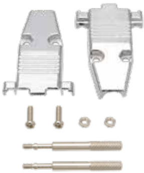
12.05.006 CAPA METÁLICA DB9/HDB15 KIT LONGO
